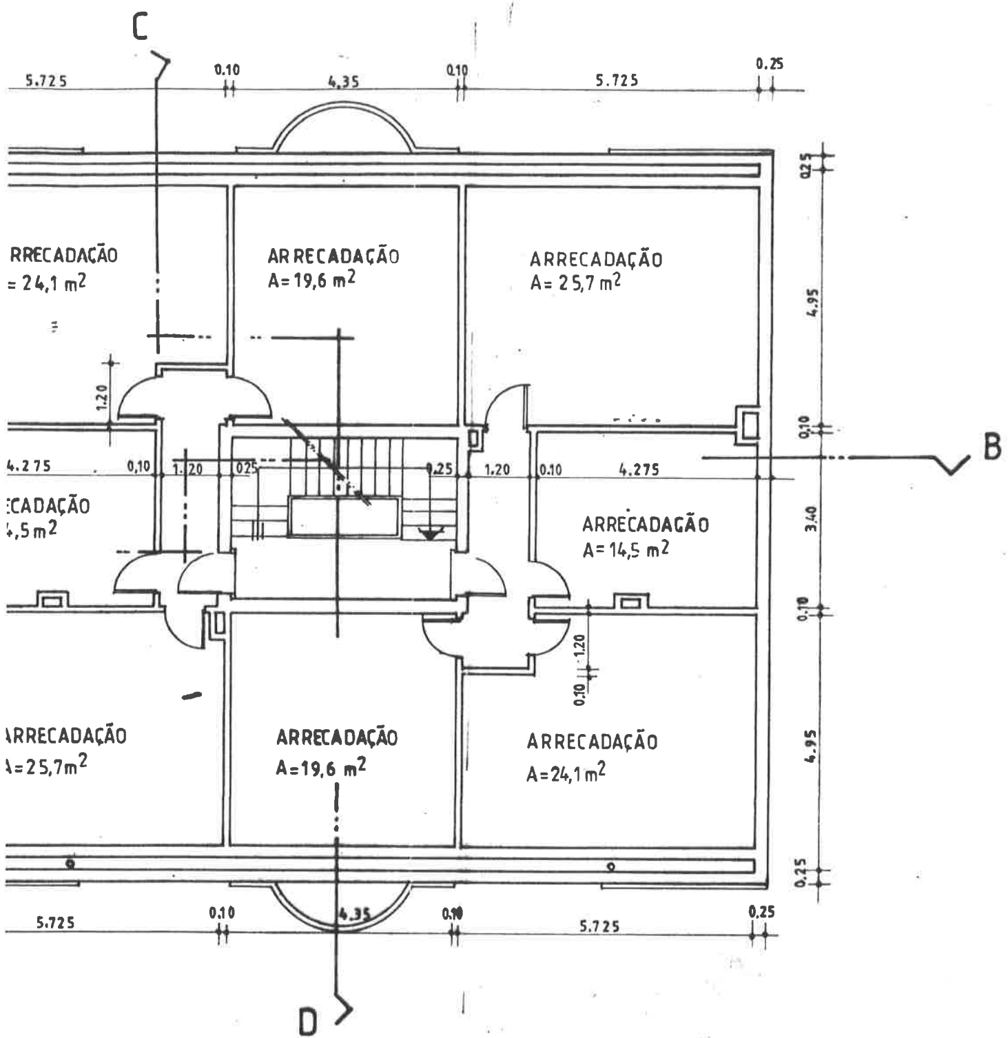
PISO 4 (Sotão)
